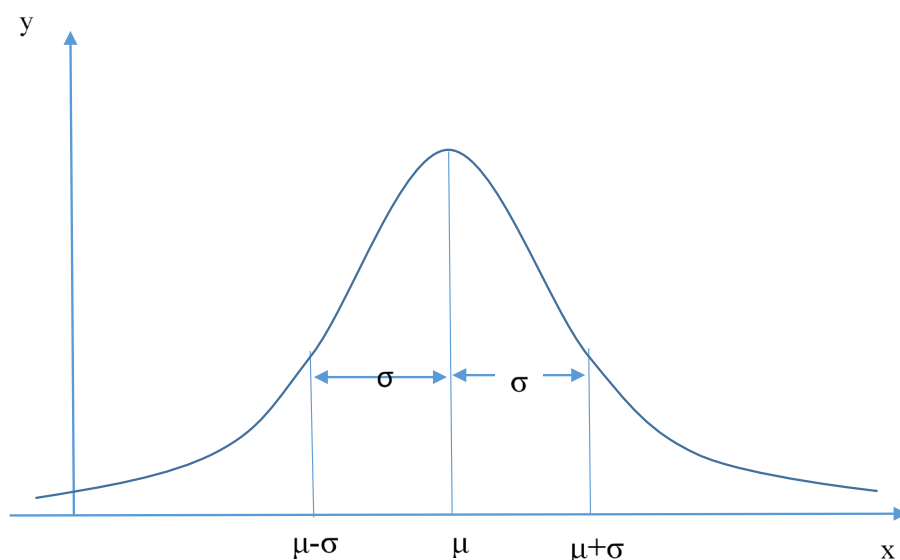
2-rasm. Normal taqsimot grafigi 2
