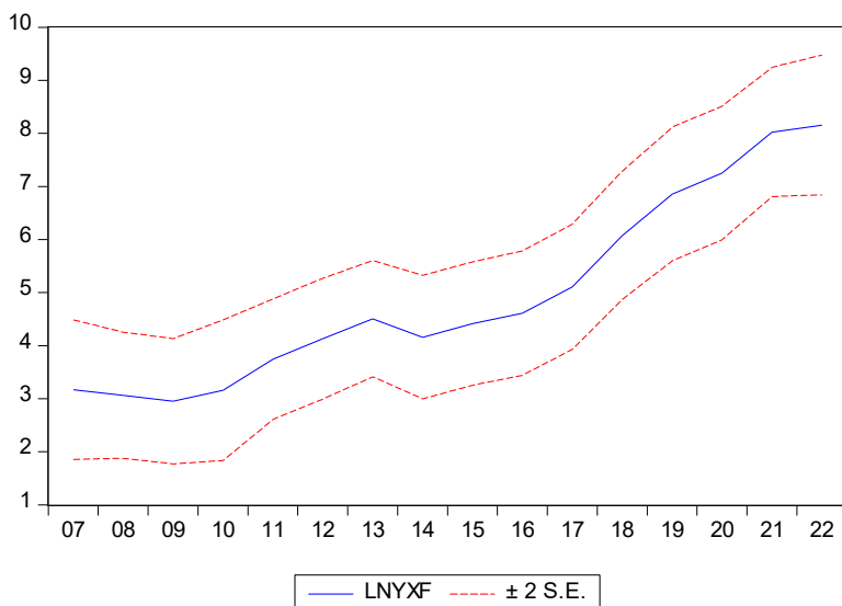
6-rasm. (2)-regressiya parametrlarini retrospektiv sifat mezonlari natijasi 6
