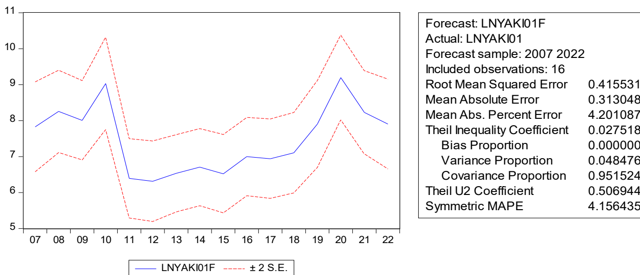
3-rasm. (1)-regressiya parametrlarini retrospektiv sifat mezonlari natijasi 3
