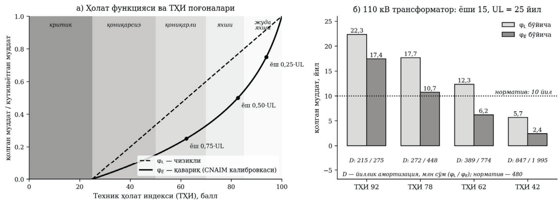
1-rasm. Holat funksiyasi (a) va 110 kV transformator misolida qolgan muddat hamda amortizatsiya (b) 3
