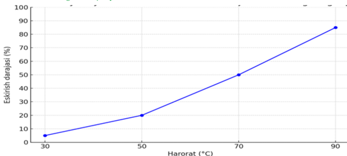
1-grafik. Kabel izolyatsiyasi harorati va eskirish darajasi o'rtasidagi bog'liqlik.
