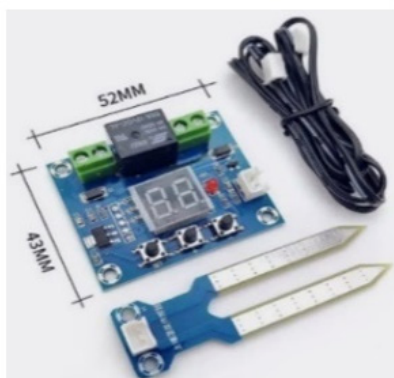
2-rasm. Namlik sensori: Tuproq namligini o'lchash DHT11 namlik sensori, pH sensori,.
