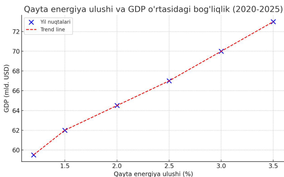
3-diagramma. Qayta tiklanadigan energiya ulushi va iqtisodiy o'sish (YAIM)
