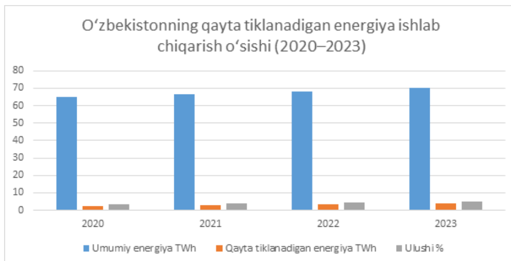
1-diagramma. O'zbekistonning qayta tiklanadigan energiya ishlab chiqarish o'sishi (2020–2023)
