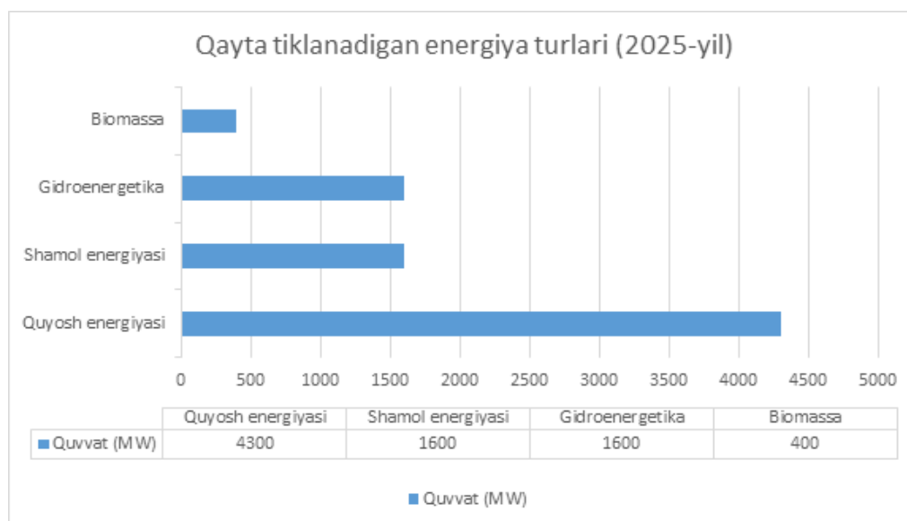
2-diagramma. Qayta tiklanadigan energiya turlari (2025-yil holatiga ko'ra) [12]
