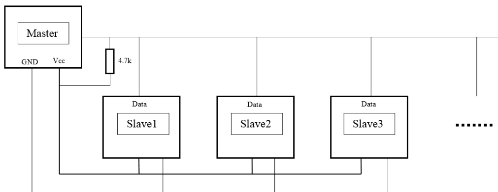
3-rasm. Bir nechta qurilmalarning 1-Wire shinasiga ulanish sxemasi
