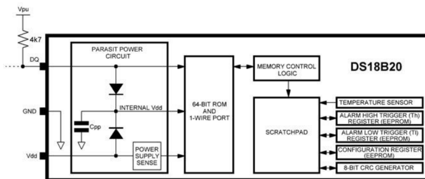
5-rasm. DS18B20 termosensorining struktura sxemasi
