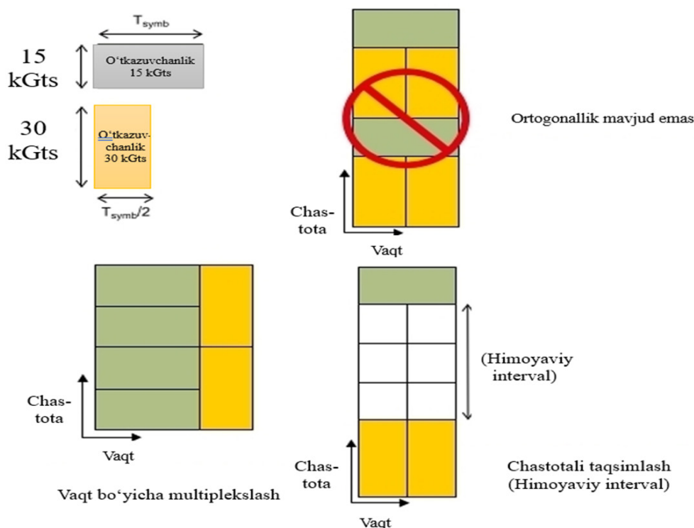
2-rasm. 30 kGts pastki tashuvchi oralig'iga ega 5G NR DSS tizimlarida shovqinlarni oldini olish uchun himoya oralig'i yoki vaqtni multiplekslash sxemasi
