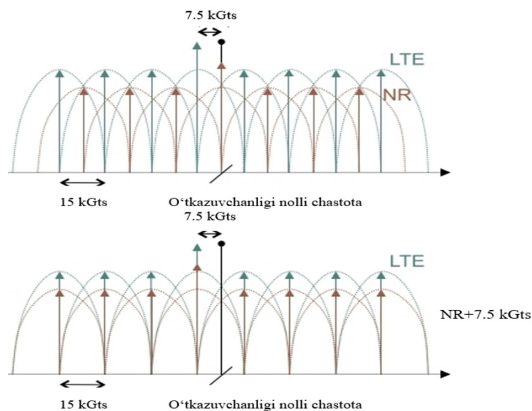
3-rasm. Yuqori oqim uzatishda 7,5 kGts chastotasini hisobga oluvchi NR texnologiyasining yangi versiyasi
