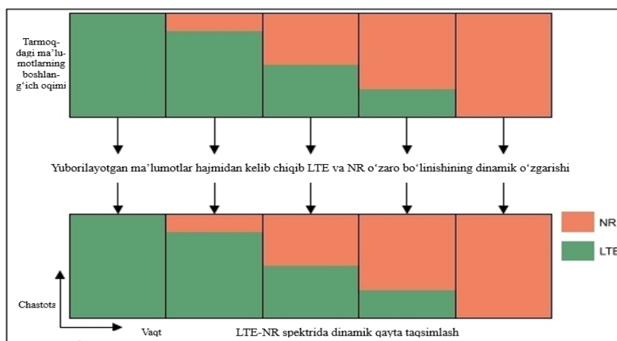
1-rasm. LTE va NR tarmoqlarining birgalikda ishlashini ta'minlaydigan chastota spektrini dinamik qayta taqsimlash konsepsiyasi
