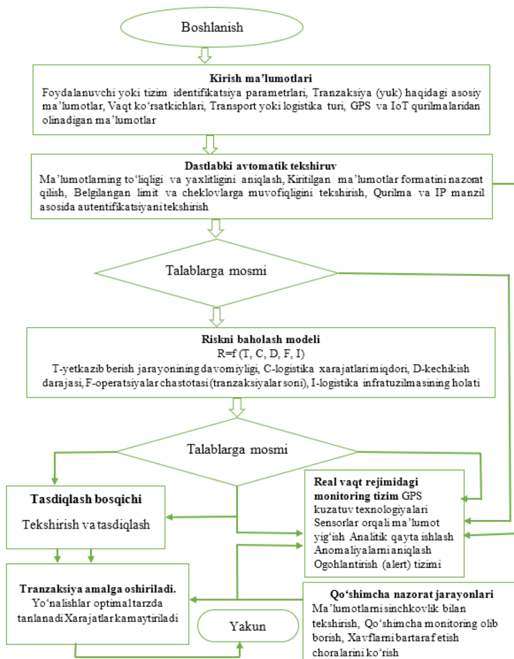
1-rasm. Kriptobirja axborot tizimida tranzaksiya so'rovlarini avtomatlashtirilgan tekshirish asosida risk baholash modeli 1
