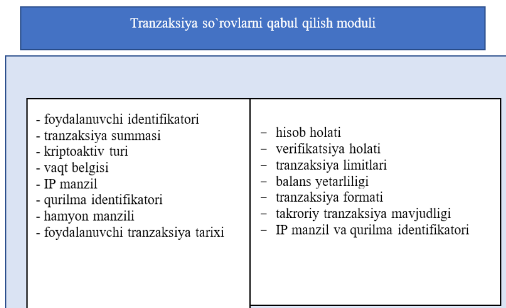
2-rasm. Tranzaksiya qabul qilish moduli 2
